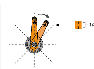
3. Sveiv ett trinn for å kompensere for sagbladet.
