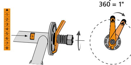
2. Sveiv en omdreining for å stille inn sagsnittet for en 1-toms planke.
