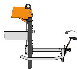
1. Trykk inn veiven for å utløse låsen.
